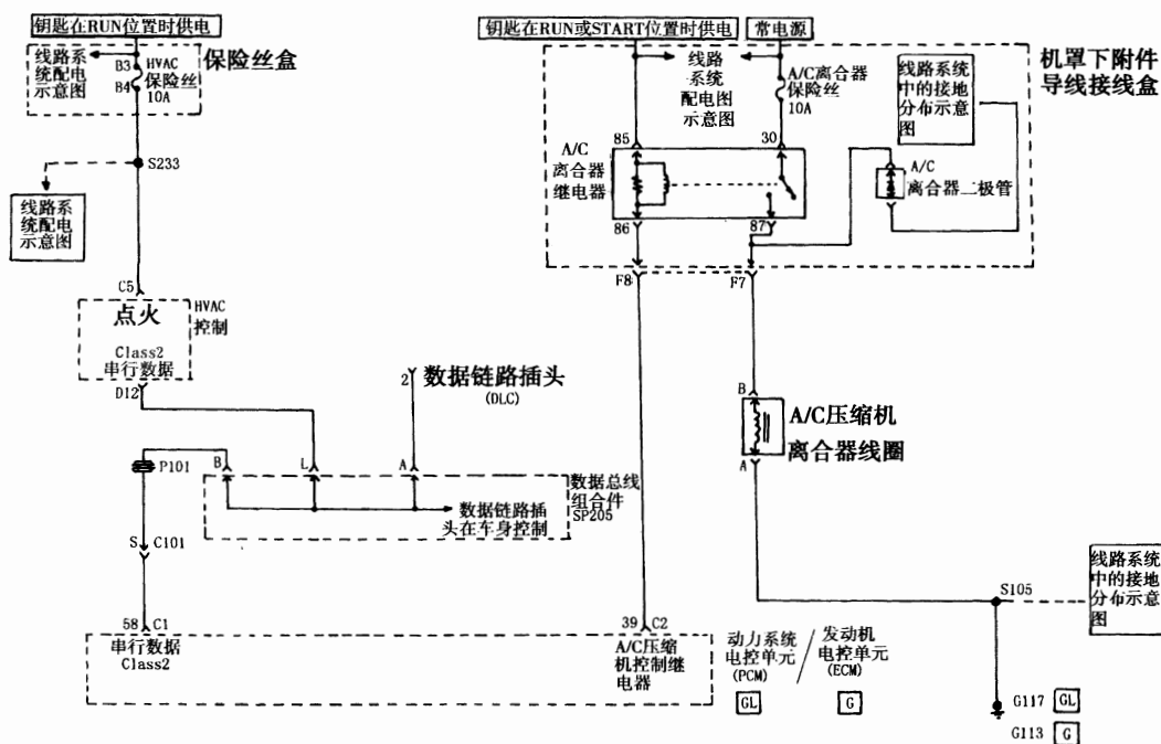
图 16—3—1 暖风、通风与空调系统压缩机控制电路图
