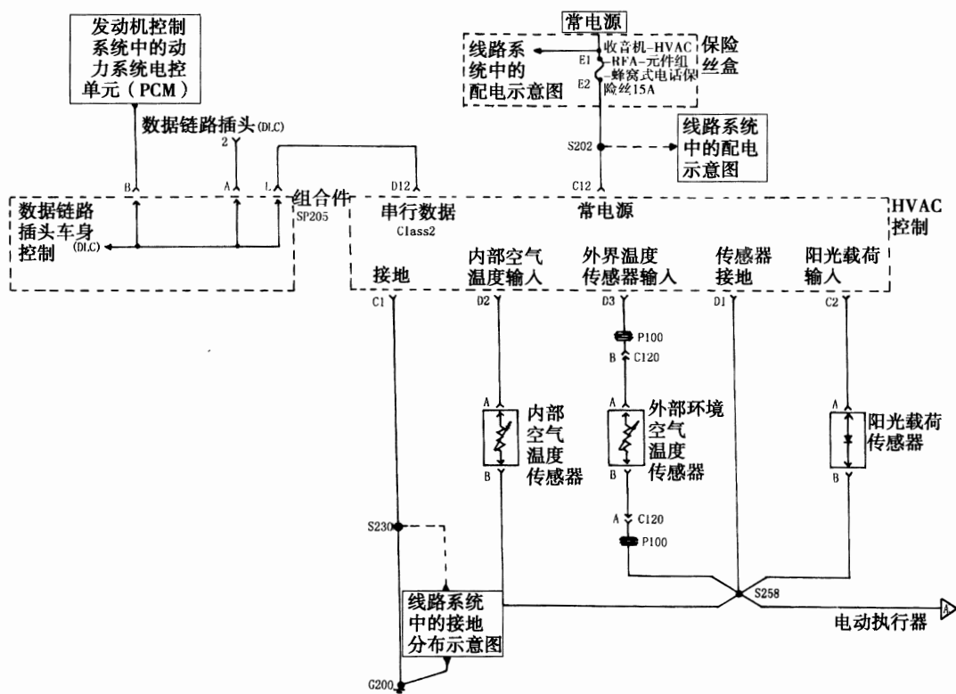
图 16—3—5 暖风、通风与空调系统空气输送/温度控制电路图①
