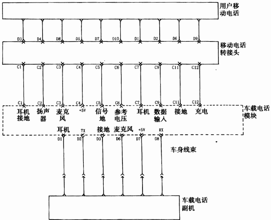
图 16—3—18 车载电话系统电路图②
