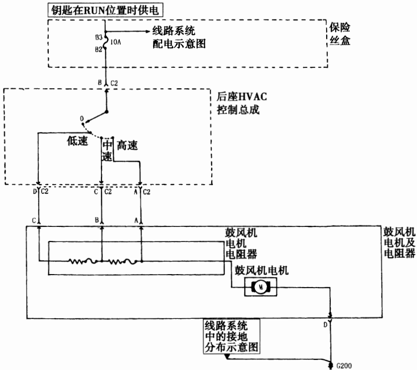
图 16—3—3 暖风、通风与空调系统鼓风机控制电路图②
