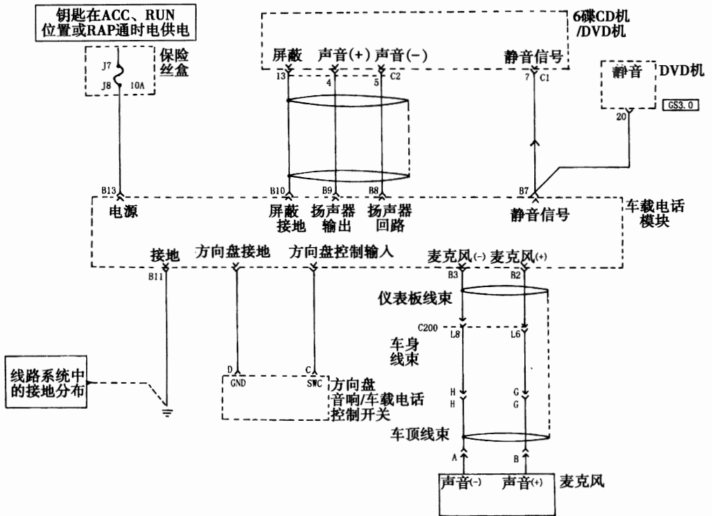
图 16—3—17 车载电话系统电路图①
