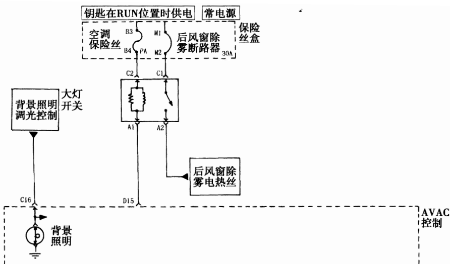
图 16—3—4 暖风、通风与空调系统鼓风机控制电路图③
