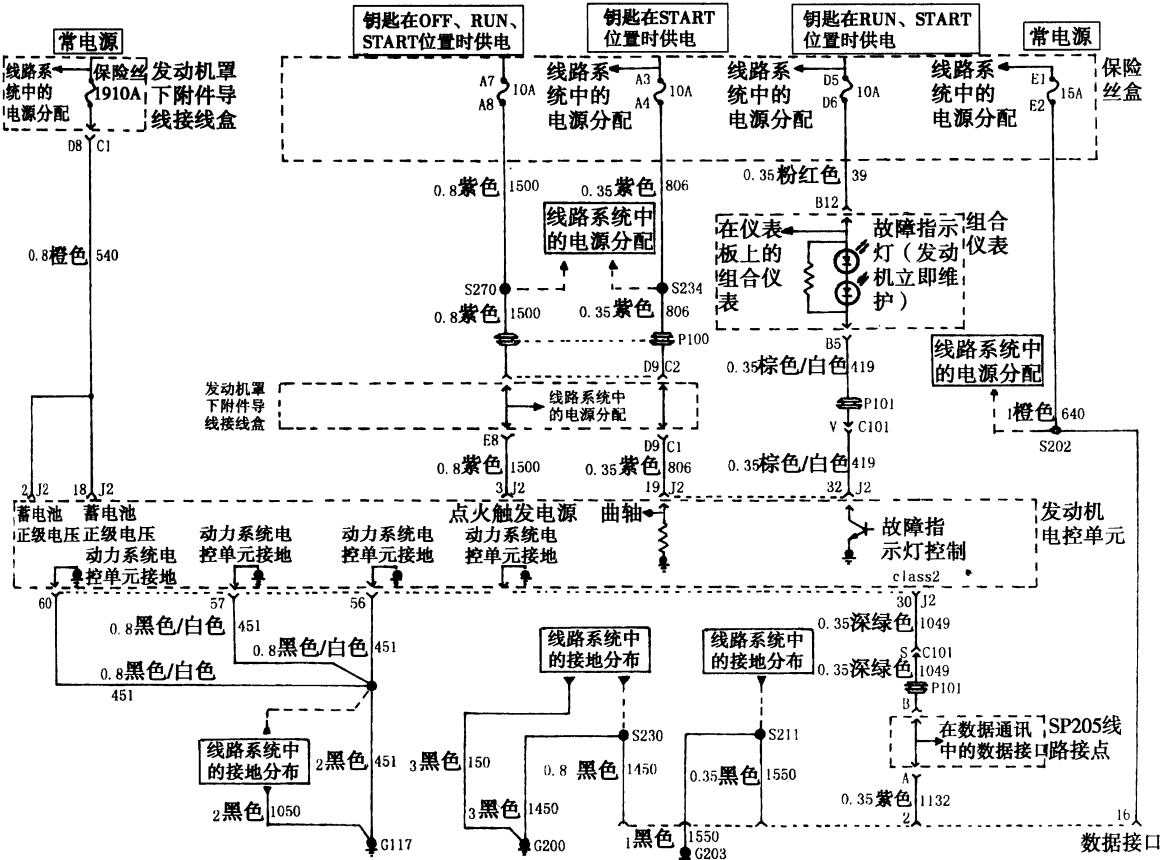
图 16—1—1 上海通用君威轿车 2.0L 发动机电路图①
