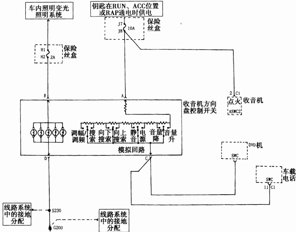
图 16—3—15 收音机/音响系统电路图⑤
