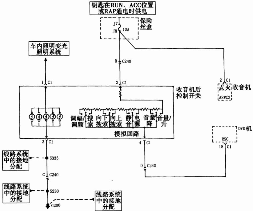
图 16—3—16 收音机/音响系统电路图⑥
