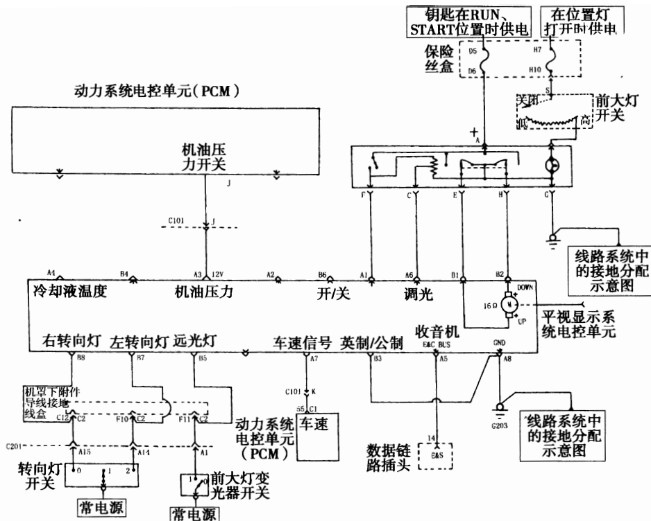
图 16—3—10 超视距抬头显示系统电路
