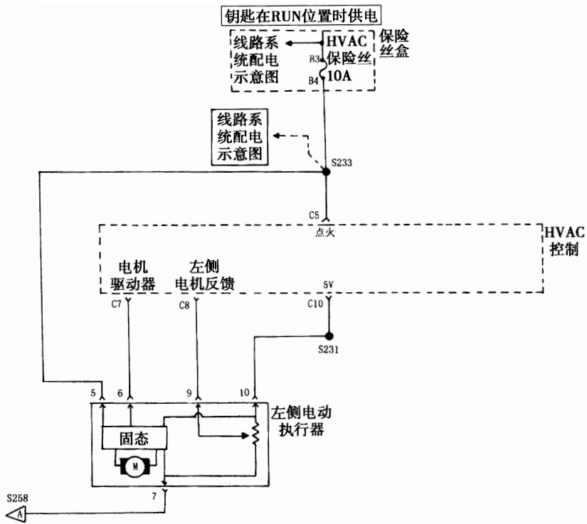
图 16—3—6 暖风、通风与空调系统空气输送/温度控制电路图②
