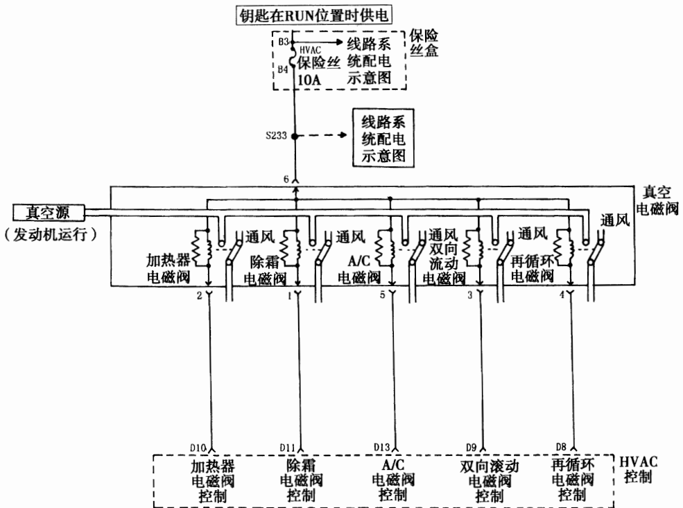
图 16—3—7 暖风、通风与空调系统空气输送/温度控制电路图③
