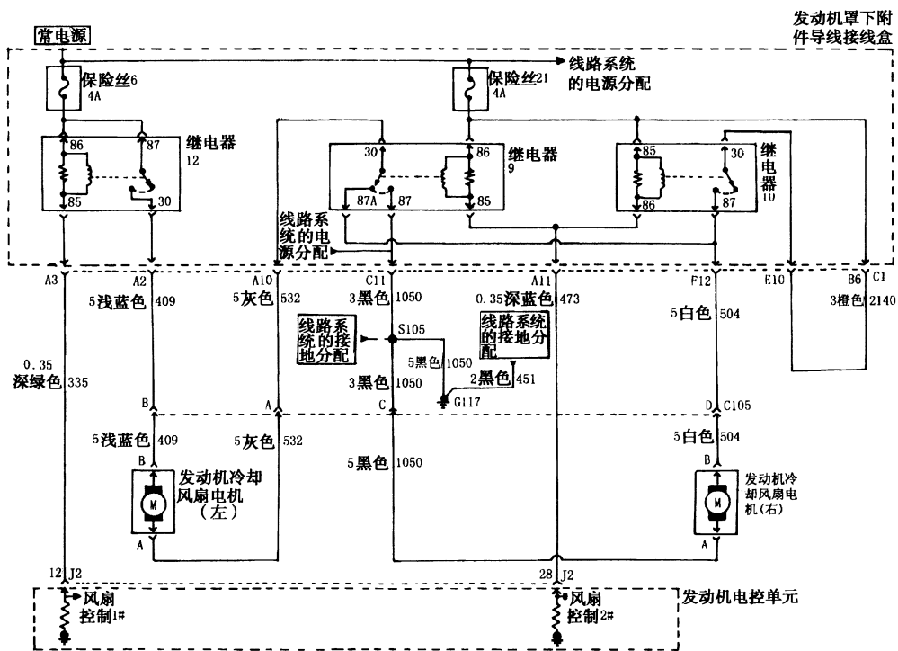
图 16—1—11 上海通用君威轿车 2.0L 发动机电路图⑪
