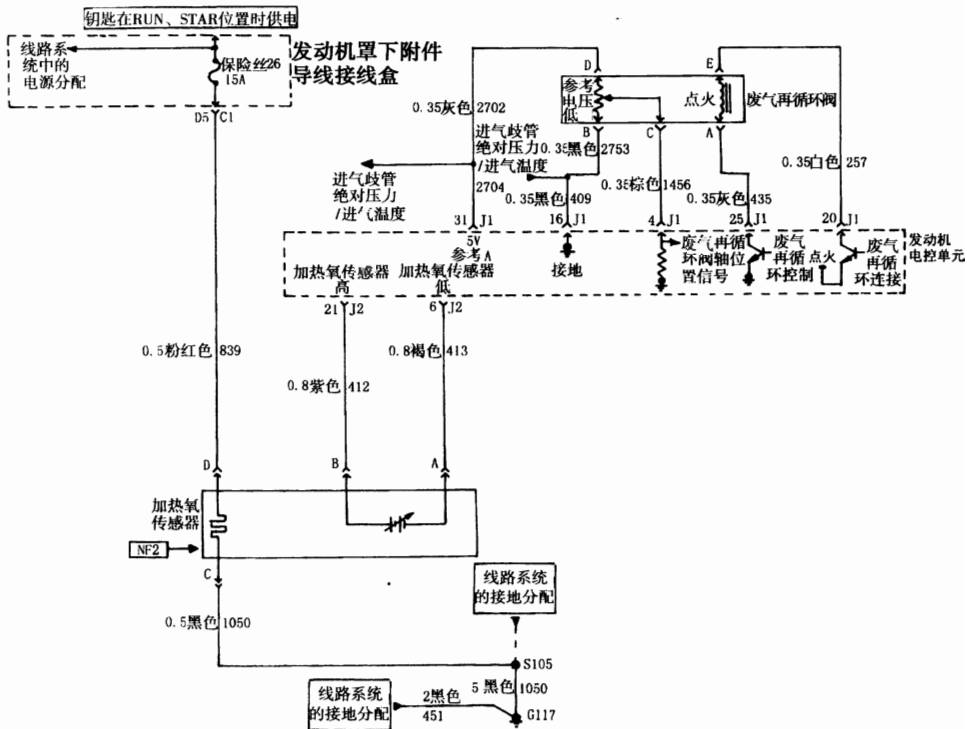
图 16—1—6 上海通用君威轿车 2.0L 发动机电路图⑥
