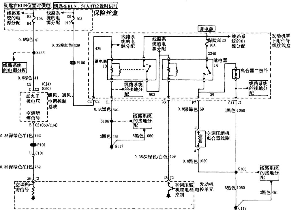
图 16—1—10 上海通用君威轿车 2.0L 发动机电路图⑩ 左右冷却风扇
