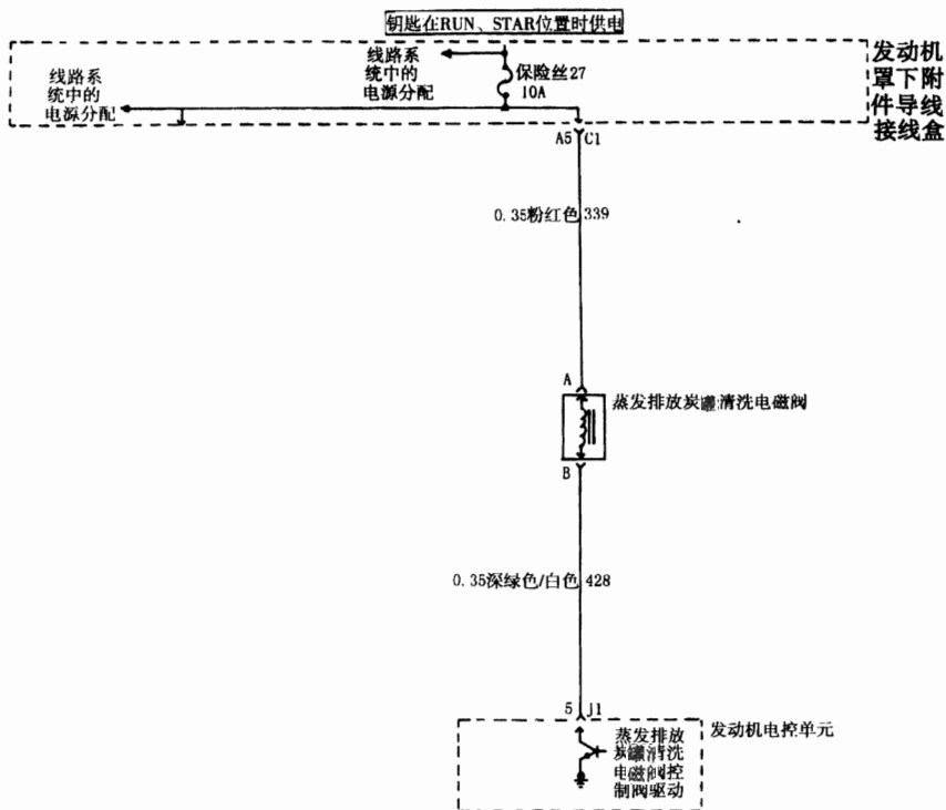
图 16—1—7 上海通用君威轿车 2.0L 发动机电路图⑦
