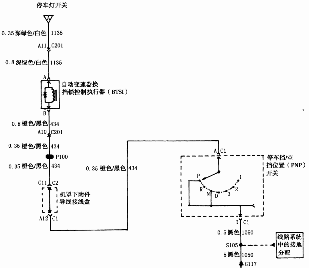
图 16-2-2 自动变速器电路图②
