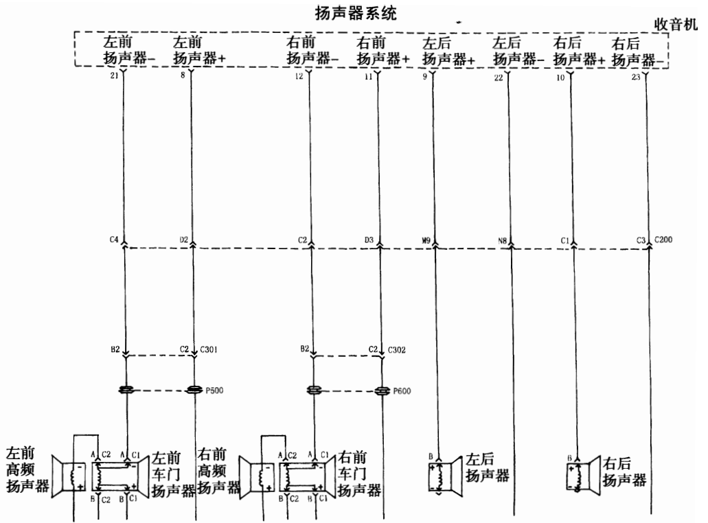
图 16—3—12 收音机/音响系统电路图② 后窗内天线和收音机天线模块
