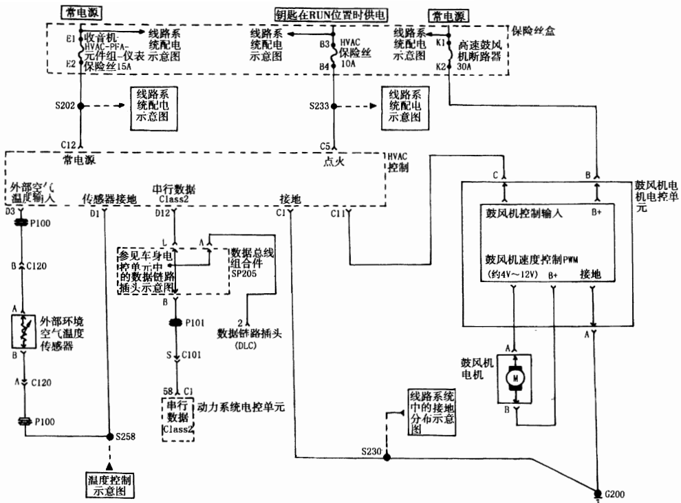
图 16—3—2 暖风、通风与空调系统鼓风机控制电路图①
