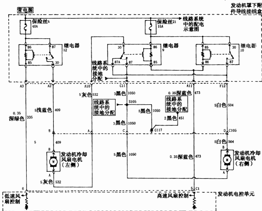
图 16—1—12 上海通用君威轿车 2.0L 发动机电路图⑫
