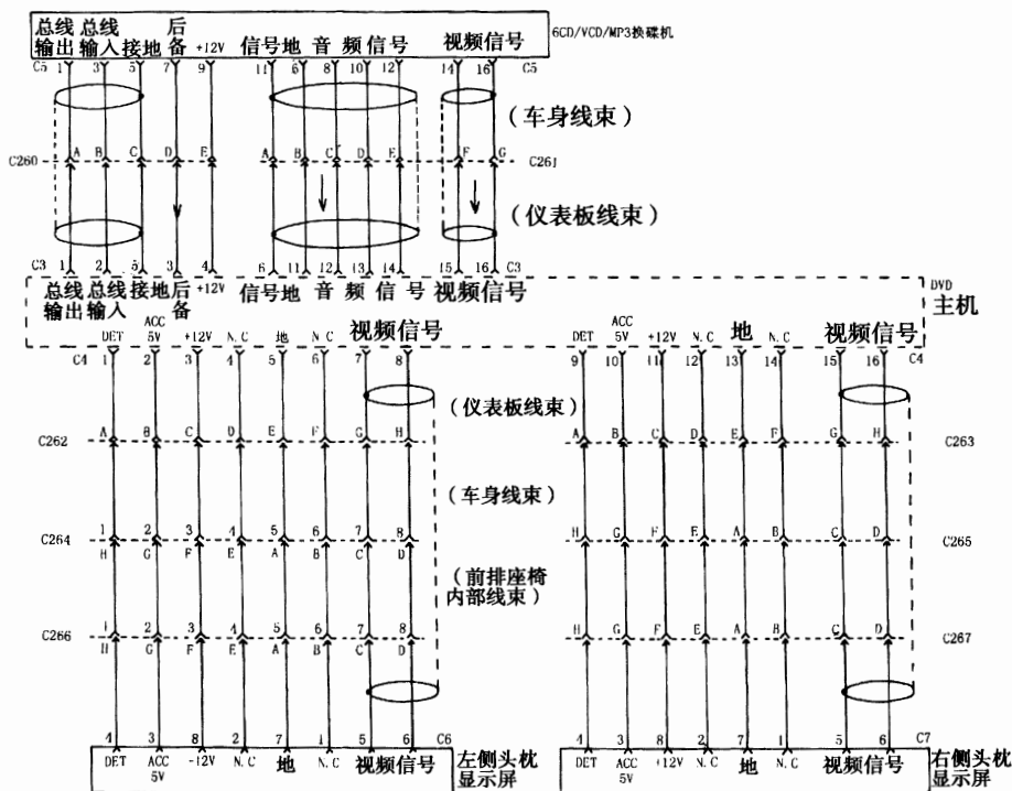
图 16—3—14 收音机/音响系统电路图④
