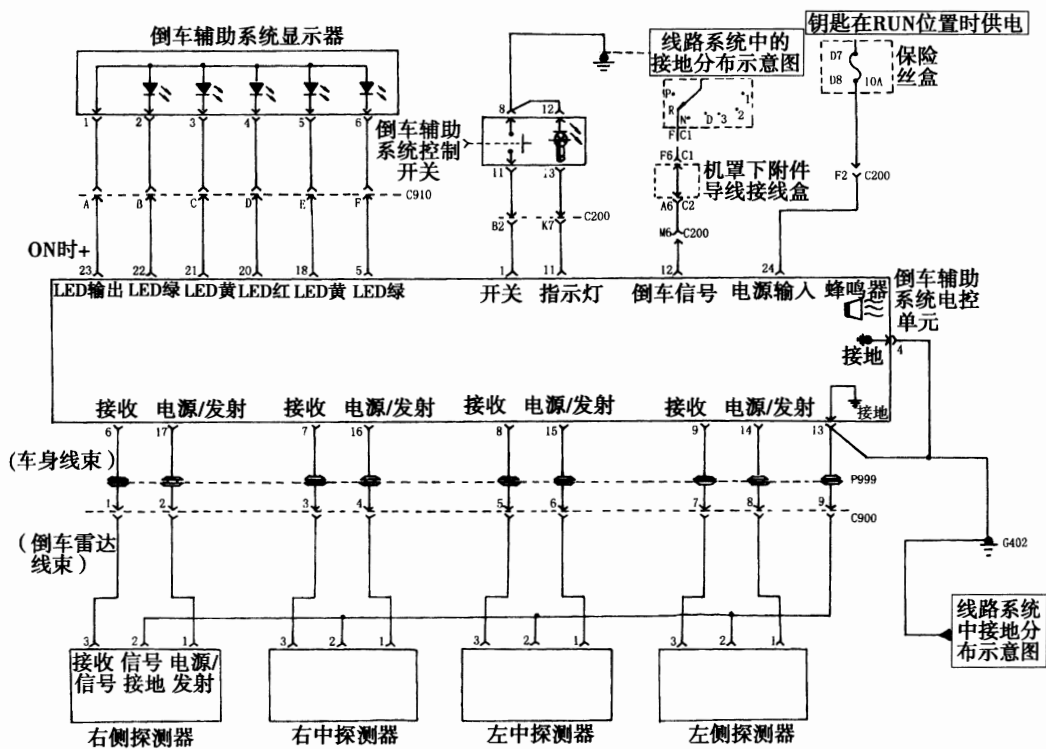
图 16—3—9 倒车辅助系统电路图
