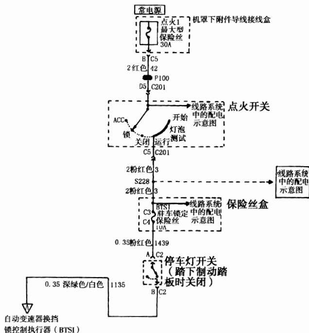
图 16—2—1 自动变速器电路图①
