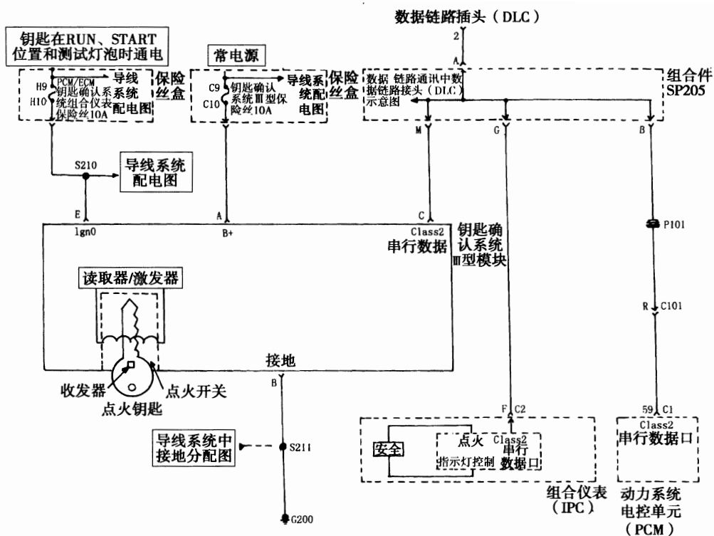
图 16—3—8 防盗系统电路图
