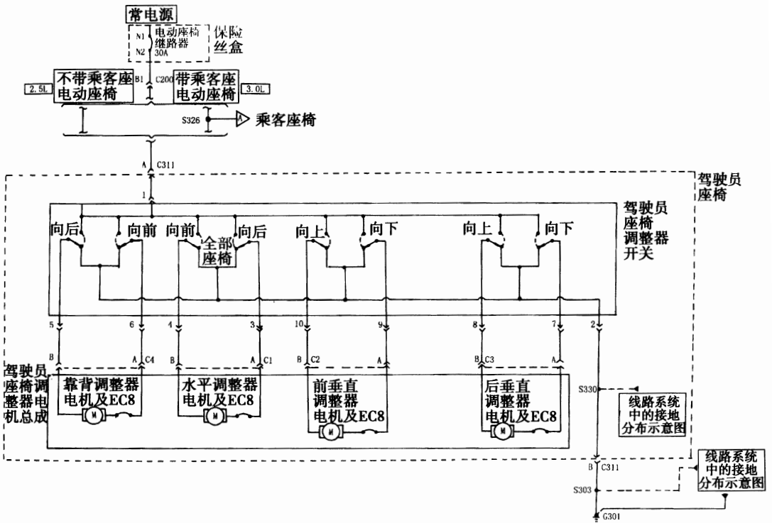
图 16—3—19 电动座椅电路图
