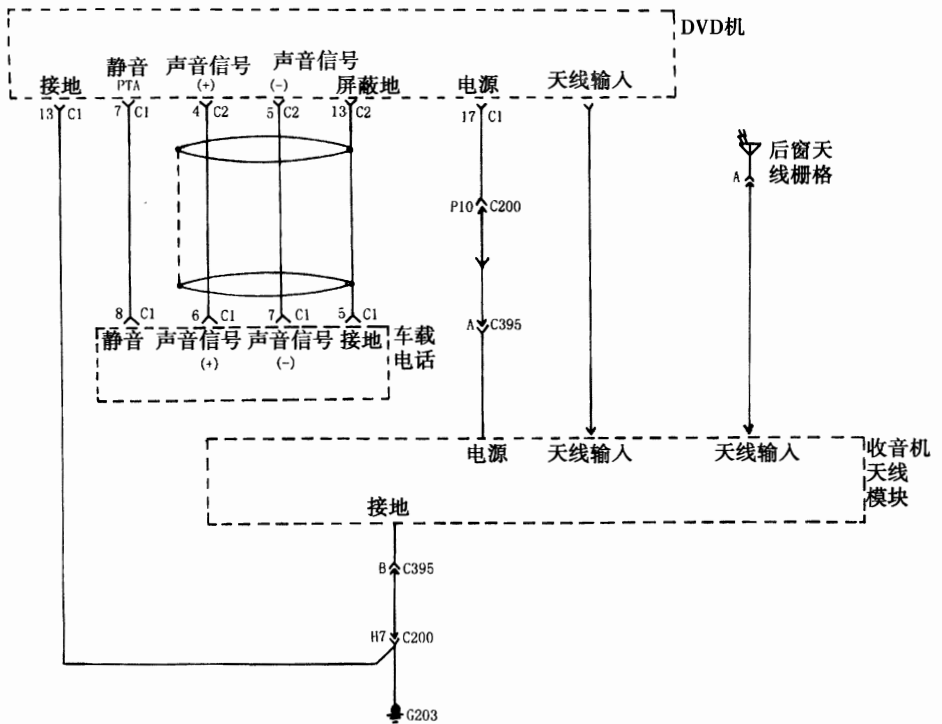
图 16—3—13 收音机/音响系统电路图③
