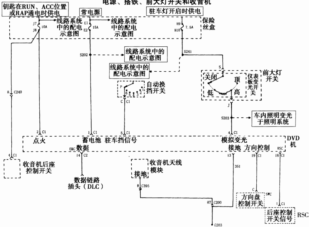
图 16—3—11 收音机/音响系统电路图①
